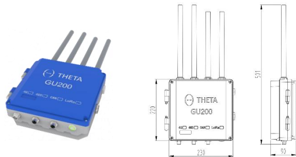
GU200-L/GU200X-L
